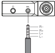
밸런스 단자 핀 배열 (2.5mm 4극)
