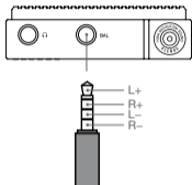
Disposition des broches du Port audio équilibré
