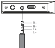
排列平衡端口插
