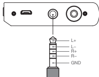
排列平衡端口插 (4.4毫米 5触点, JEITA 标准规格)
