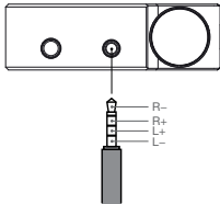
밸런스 단자 핀 배열 (2.5mm 4극)
