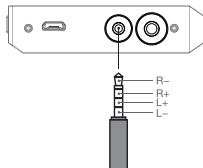
バランス端子ピン配列
